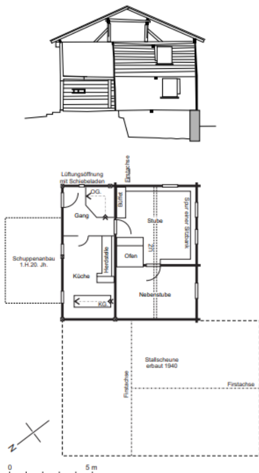
Abb. 6: Grundriss Erdgeschoss du Querschnitt, 1:200.
