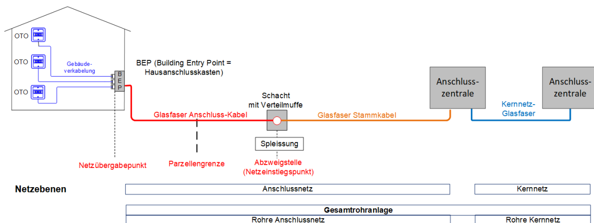
Abbildung 14 Kabelkanalisation: Schema
