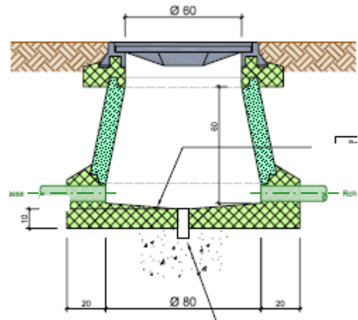
Abbildung 10 Kabelkanalisation: Kontrollschacht
