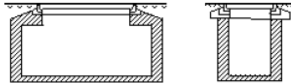
Abbildung 7 Kabelkanalisation: Kleineinstiegschacht
