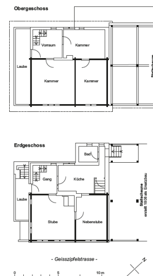
Abb. 3: Grundrisse 1:200.
