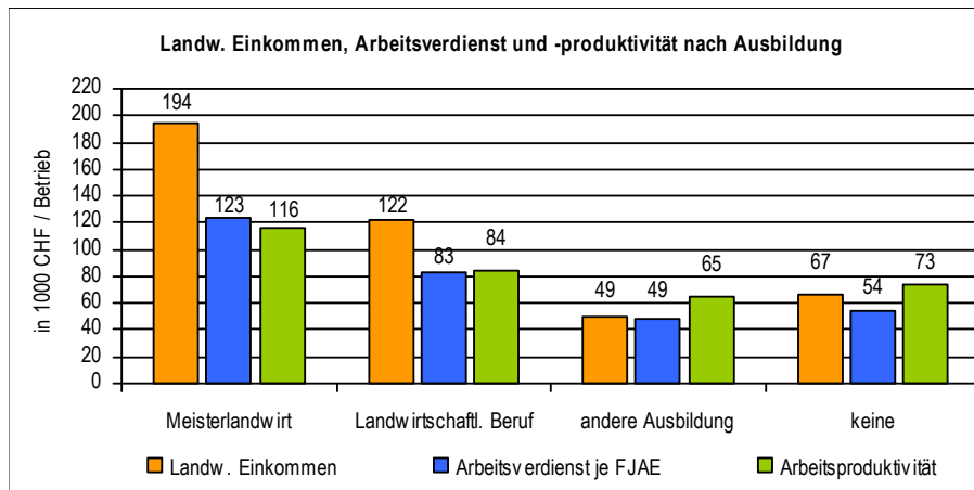
Abbildung 94: Landwirtschaftliches Einkommen und Arbeitsverdienst nach Ausbildung 2008
