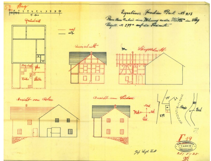
Abb. 2: Projektplan 1925 zum Bau eines Wohnhauses für unverheiratete Grenzwächter.
