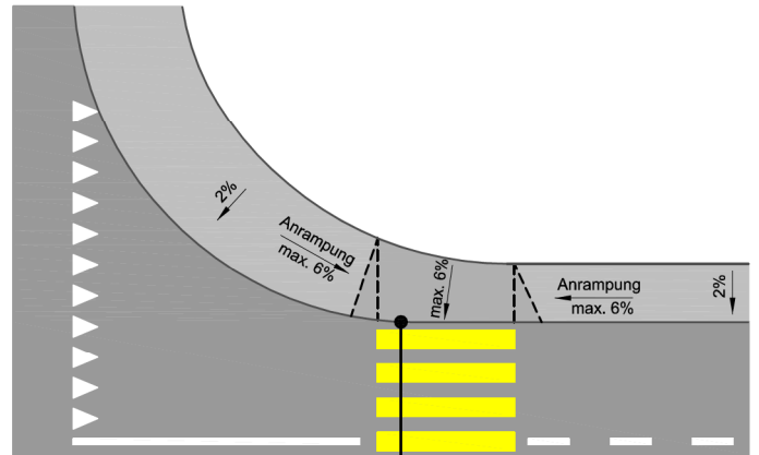
Detail Trottoirabsenkung
