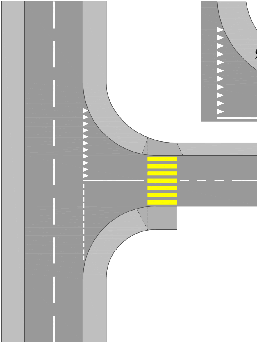
Detail Trottoirabsenkung
